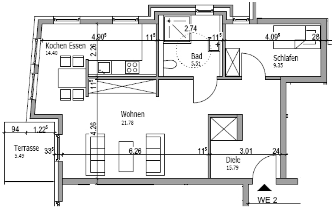
Wohnbeispiel 2
